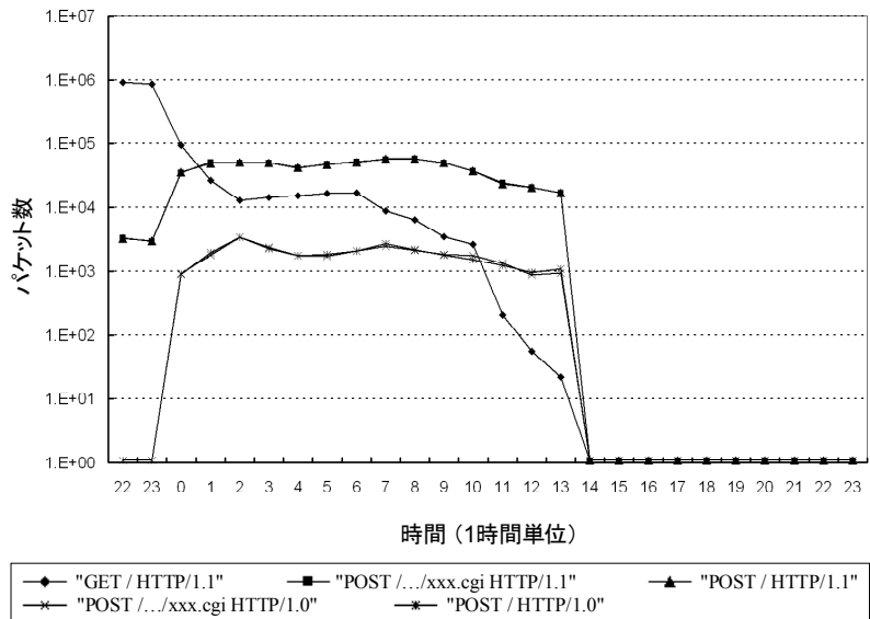
図 3 観測日 A2(ゾロ目の日)の HTTP メソッド別パケット数推移
