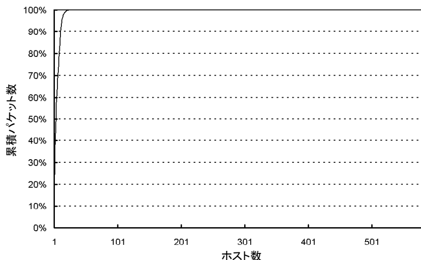
図 4 観測日 B1 (観測月の 1 日)の“GET / HTTP/1.1”
