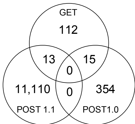
図 8 攻撃手法の重複
