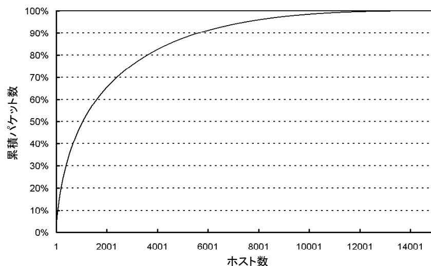
図 7 観測日 B3 (観測月のゾロ目の日)の“POST / HTTP/1.1”
